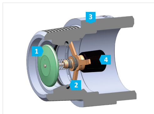
SENTRY GS Schnittmodell (DN25)
