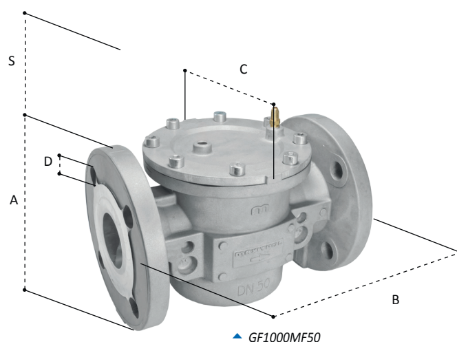
▲ GF1000MF50
